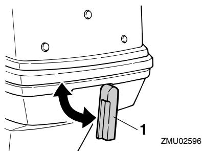
1. Рычаг(и) замка верхней части кожуха
